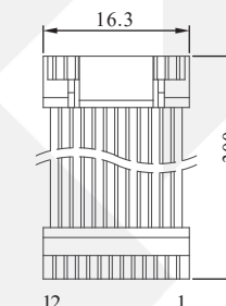
Cable: YCW047
